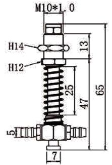
TL-M10-L65-7
