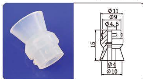
CP-10DS
