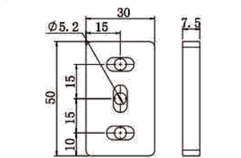
3050平面光滑夹片
