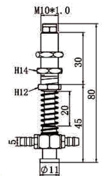
TL-M10-L80-11B
