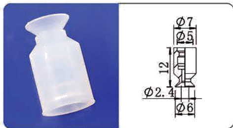
CP-6
