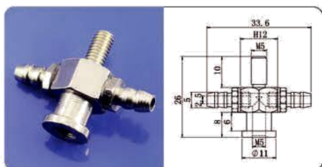
大头M5外牙气缸头
