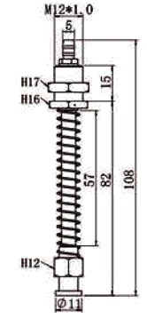
TS-M12-L108-11
