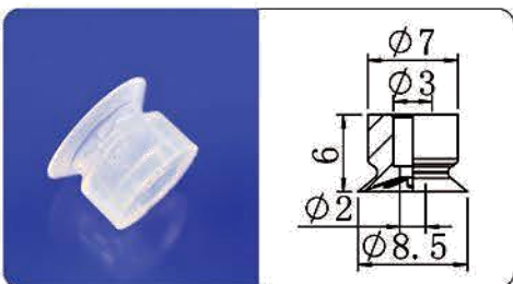
CP3-08UM
