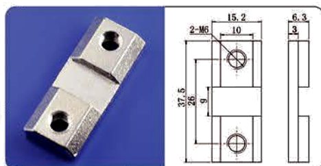
两孔螺母02-M6
