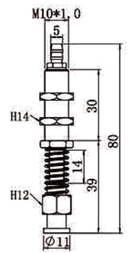
TS-M10-L80-11B
