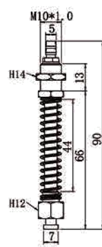
TS-M10-L90-7
