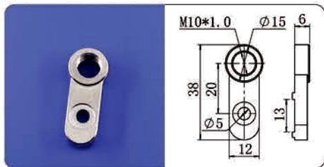
精锐固定块M10
