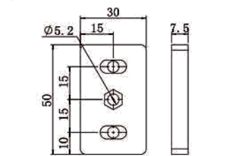
3050平面防滑夹片
