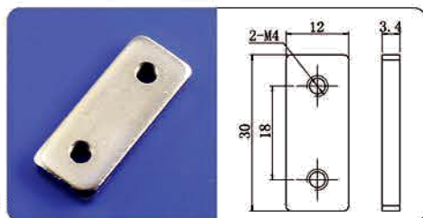
两孔螺母M4
