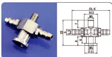
M5气缸头牙短
