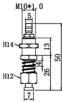
TS-M10-L50-7
