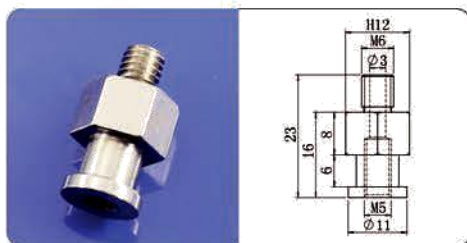
大头金具转换头HSPPS-M6
