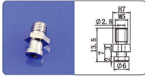
M5微型金具PS专用
