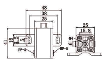
MCD-10大角抱具
