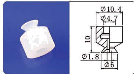
SP-6
