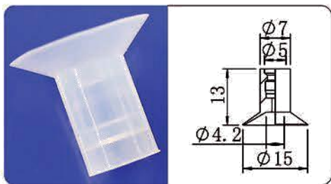
CP-15
