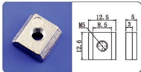
哈模单孔螺母(海尔精锐)
