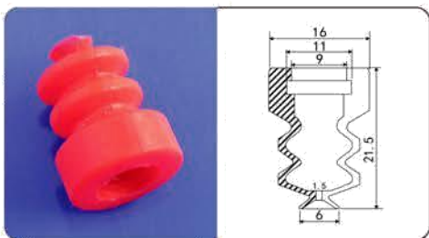
YX-6-3R
