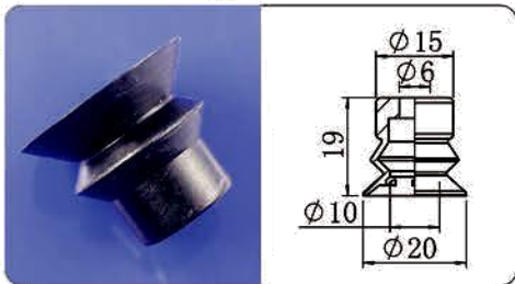
VP-20B
