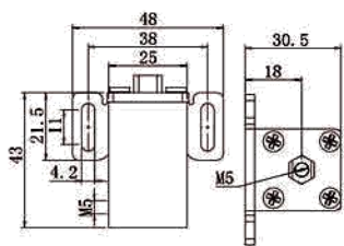
1815抱具气缸(扁六角)
