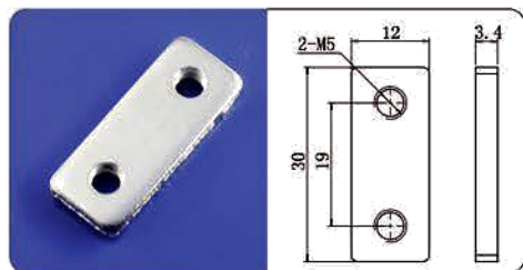
两孔螺母M5
