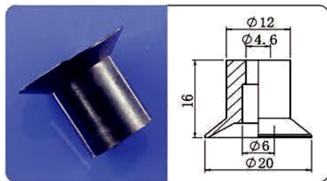
H-20N
