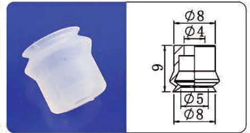
PJG-8
