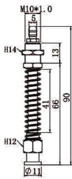
TS-M10-L90-11
