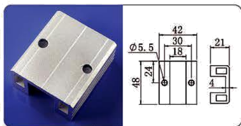
单槽通孔固定块
