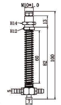
TL-M10-L100-7
