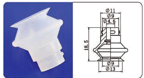
CP-13B
