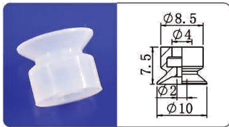
PF-10
