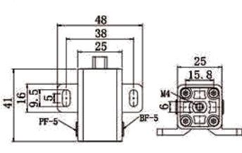
MCD-10椭圆杆抱具
