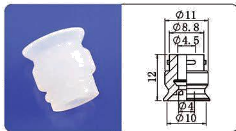
CP-10CS
