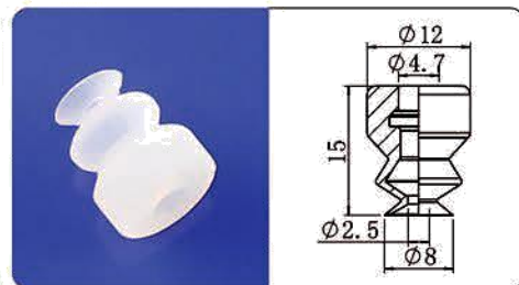
SP-8-2
