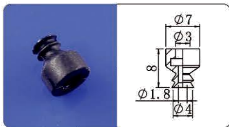
CP3-04BN
