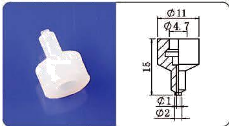
SPL-2
