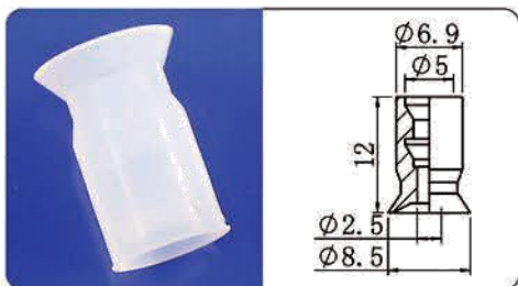
CP-08U
