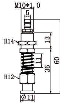
TS-M10-L60-11
