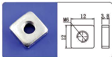
单孔螺母M6
