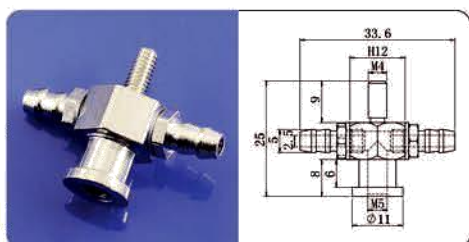
大头气缸转换头M4
