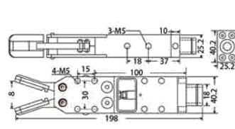
斜臂式
