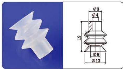
PC-13
