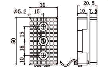
3050椭圆防滑检知抱片
