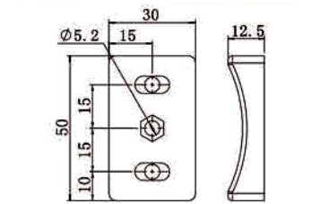
3050半圆光滑夹片
