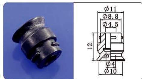
CP-10CN
