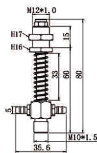
M10-M12-L80 1.5粗牙
