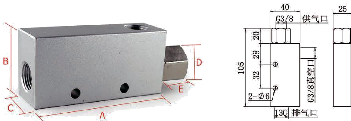
CV-20PT标准型真空发生器
