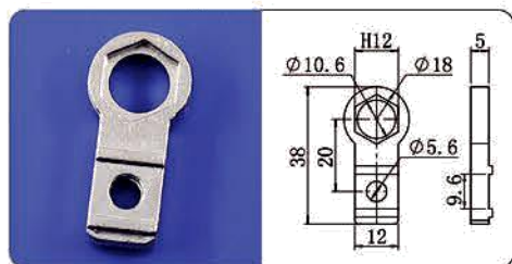
小头M10固定块
