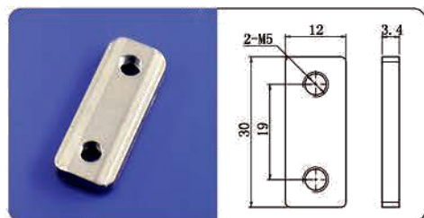
压铸两孔螺母M5
