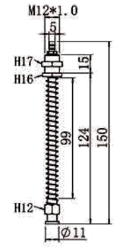
TS-M12-L150-11
