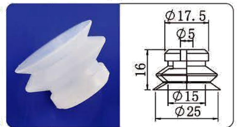
PJG-25
