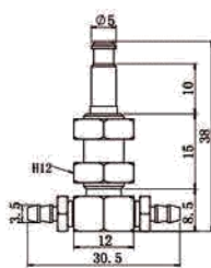
T-M8-L38尖头(镀镍)
