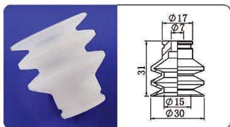
SR-30-3S
