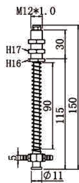
TL-M12-L150-11B
