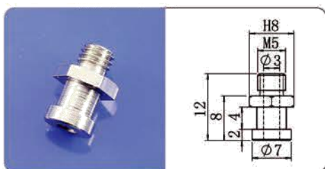
小头金具转换头SPPS-M5
