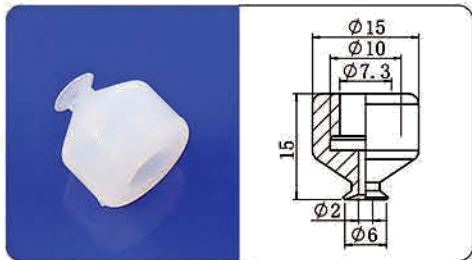
HSP-6 白色(S)
