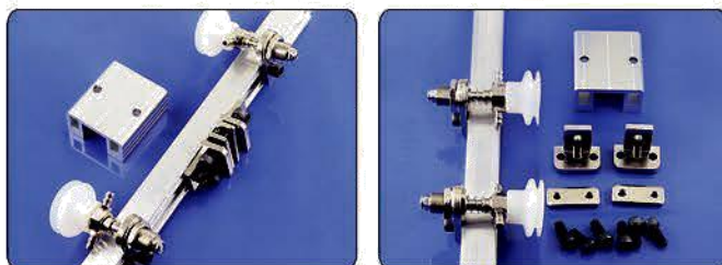
铝条固定块配件
