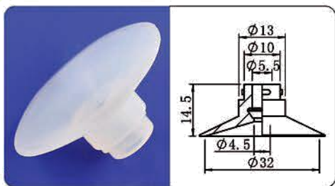
CP-32U
