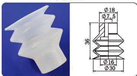
PC-30
