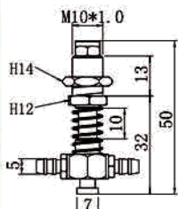
TL-M10-L50-7
