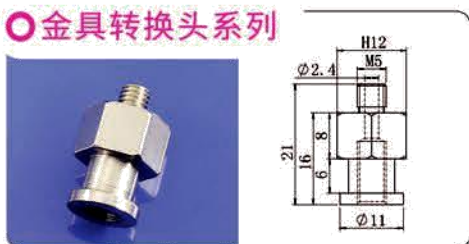
HSPPS-M4外牙M5内牙
