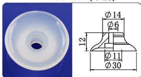
PF-30
