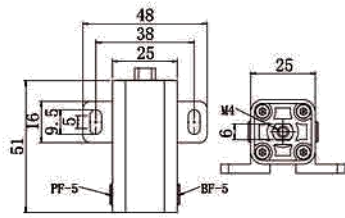
MCD-20大角抱具
