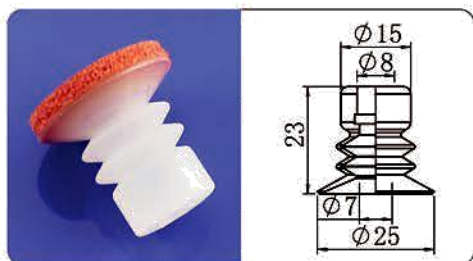
无痕HSP-25-3
