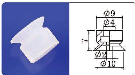
CP3-10UM
