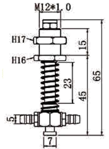
TL-M12-L65-7
