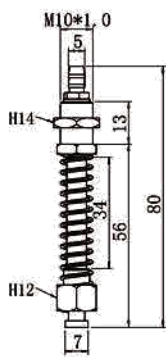
TS-M10-L80-7
