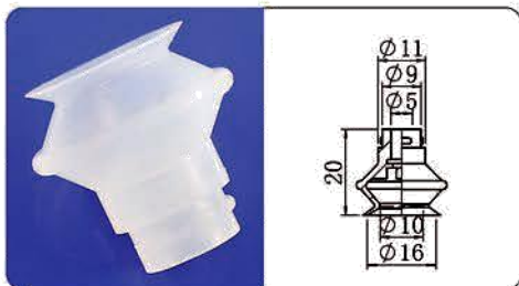
CP-16B
