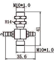
M10-M10-L43 1.0细牙
