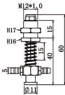
TL-M12-L60-11K
