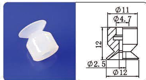
SP-12
