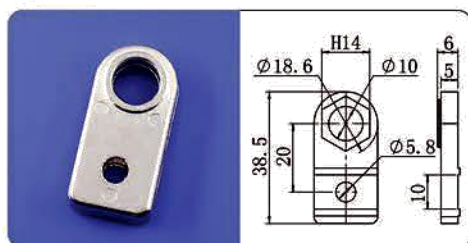
天行金具固定块M10
