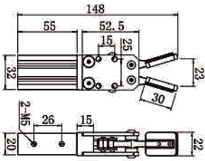
JZ1615D双动
