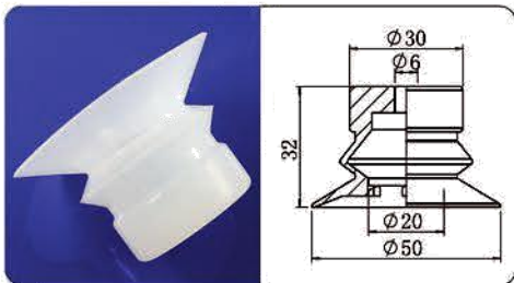
VP-50B
