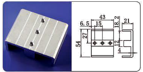
双槽通孔有牙M5铝条固定块
