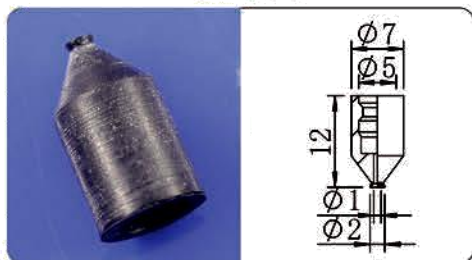
CP-2N
