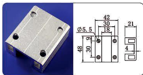
单槽通孔(四个孔)
