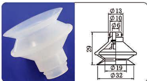
CP-32B
