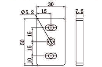
3050N平面防滑夹片
