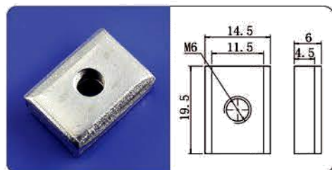
单孔长方形螺母M6
