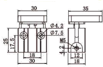
1205PT抱具
