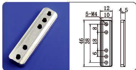
五孔螺母M4
