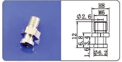
小头金具转换头M6
