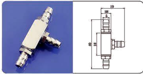
三通气咀转换头
