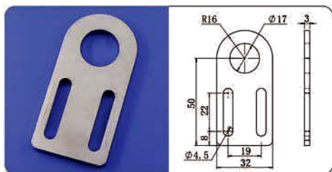
金具固定板B-17
