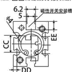
MHZ2-□□ 的磁性开关安装槽尺寸
