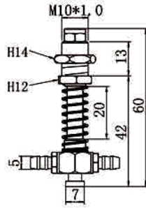
TL-M10-L60-7
