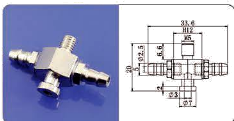
小头气缸头M5外牙
