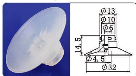
CP-32C
