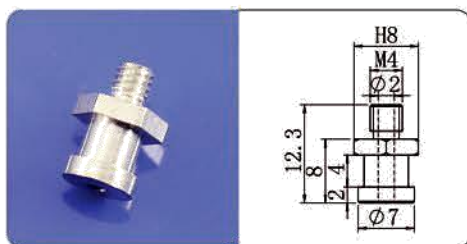
小头金具转换头SPPS-M4
