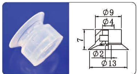
CP3-13UM
