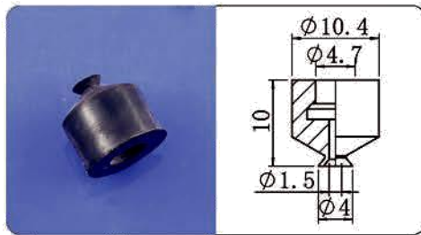
SP-4 黑色(N)
