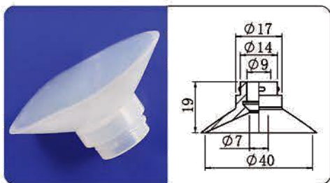
CP-40U
