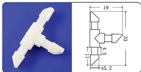
无牙塑料三通接头#6
