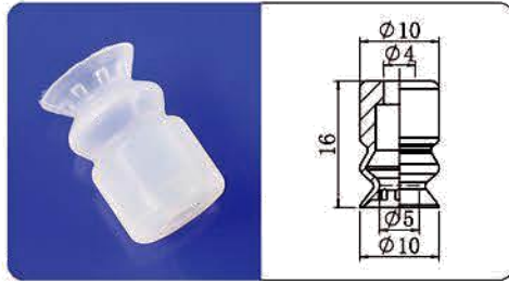
VP-10B
