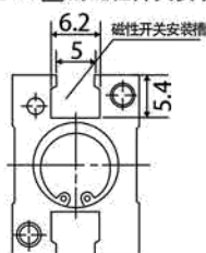
MHZ2-10□ 的磁性开关安装槽尺寸
