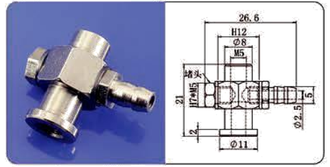
M5内牙气缸头(单侧通)
