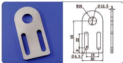
金具固定板B-12.5
