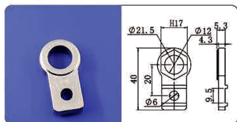
天行金具固定块M12
