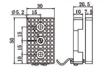
3050椭圆防滑检知抱片
