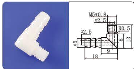
有牙塑料弯头M5
