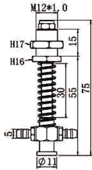
TL-M12-L75-11
