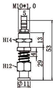
TS-M10-L53-11K
