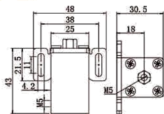
1815抱具气缸(椭圆)
