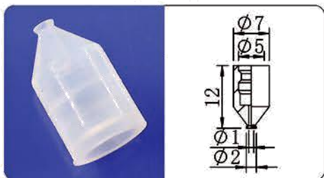
CP-2S
