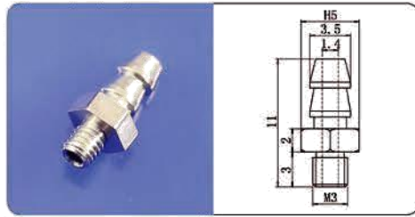
M3-4二节气咀
