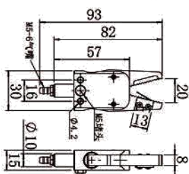
Mini-A内牙带检知
