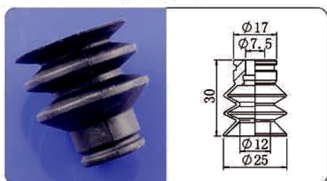
SR-25-3N
