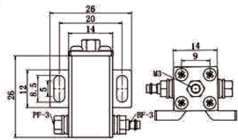
UMCD-10六角杆抱具
