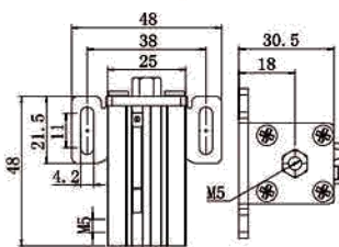
1815CH抱具(带磁)
