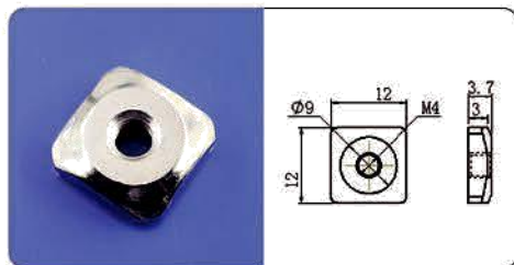
单孔螺母M4
