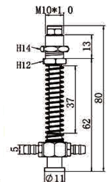
TL-M10-L80-11
