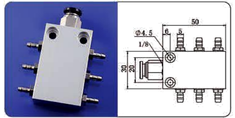
1分6气排
