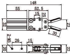
JZ1615S单动
