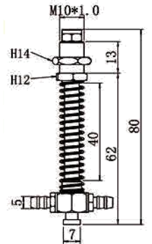
TL-M10-L80-7
