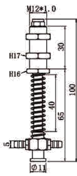
TL-M12-L100-11B
