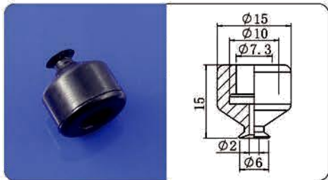
HSP-6 黑色(N)
