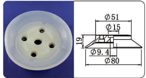
CP-80H
