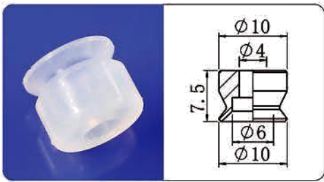
VP-10R
