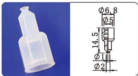
CPL-2
