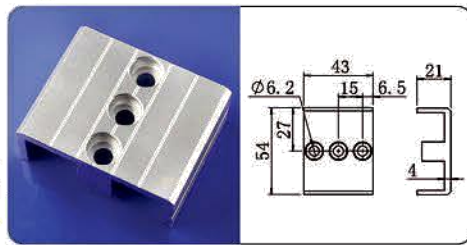
双槽通孔铝条固定块
