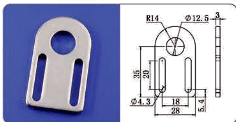
金具固定板A-12.5
