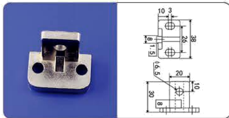
天行治具大L块
