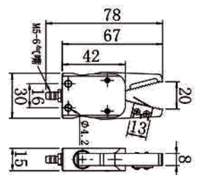
Mini-C带检知
