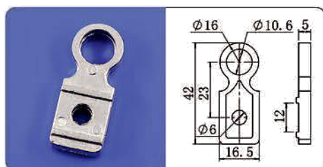
金爪
