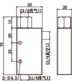
CV-15PT标准型
