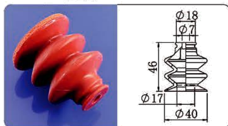
星塔无痕SR-40-3
