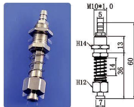
TS-M10-L60-7K
