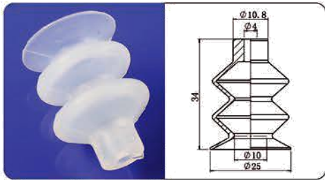
H-25-3
