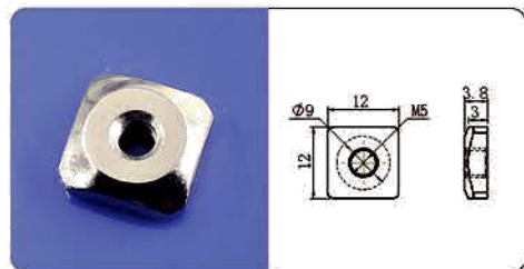
新款单孔螺母M5
