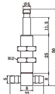
T-M8-L50尖头(镀镍)
