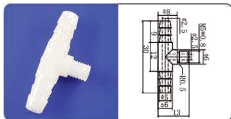
有牙塑料三通接头M5
