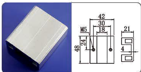
单槽M5不通孔
